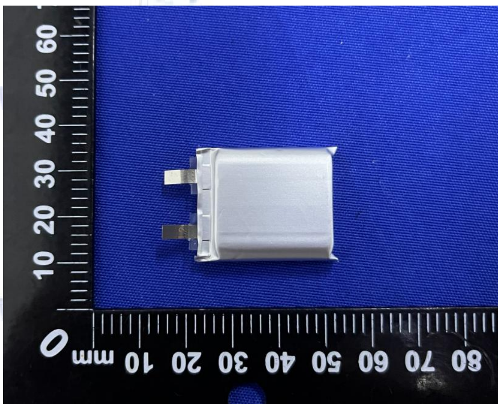
Photo 4 内部电芯 Internal Cell
